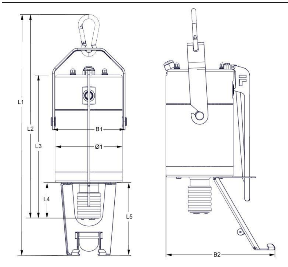
Рис. 3-3 Электродвигатель TM-E6000_evo3
