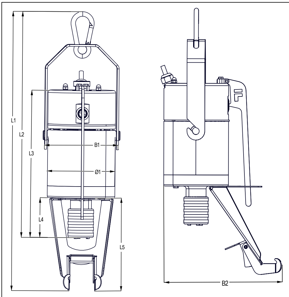
Abb. 3-5 Электродвигатель MDL1
