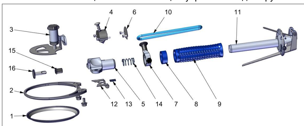
Рис. 3-1 Trimmer 128_evo3 (Пример)
