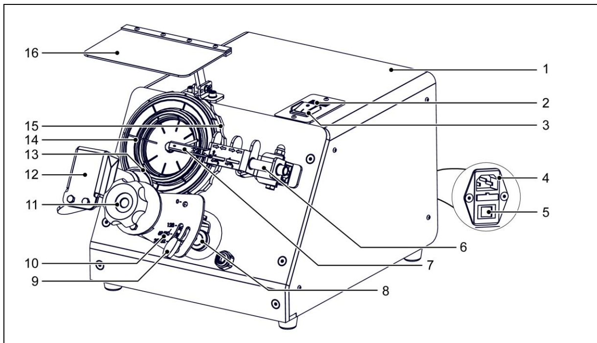
Рис. 3-7 Вид TSM-E1
