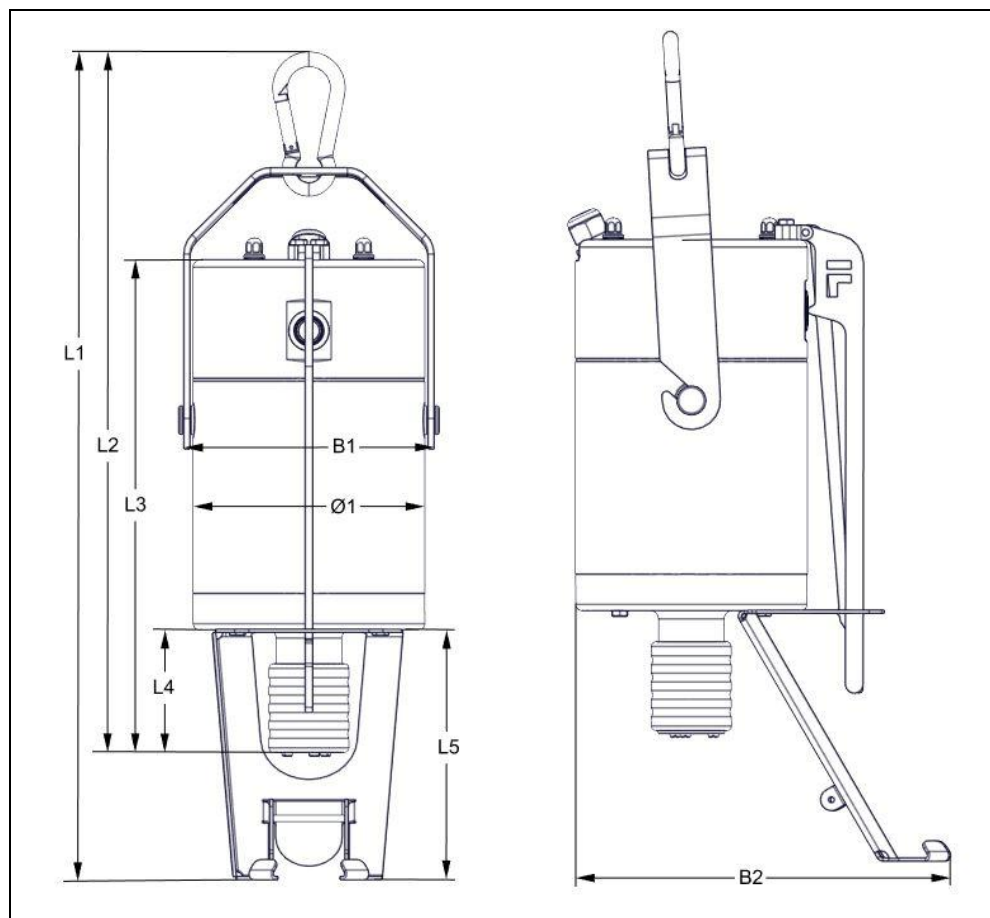
Rys. 3-3 Motor TM-E6000_evo3
