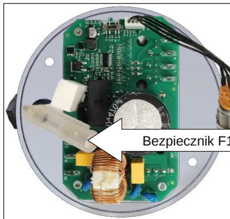
Abb. 8-1 Umiejscowienie bezpiecznika
