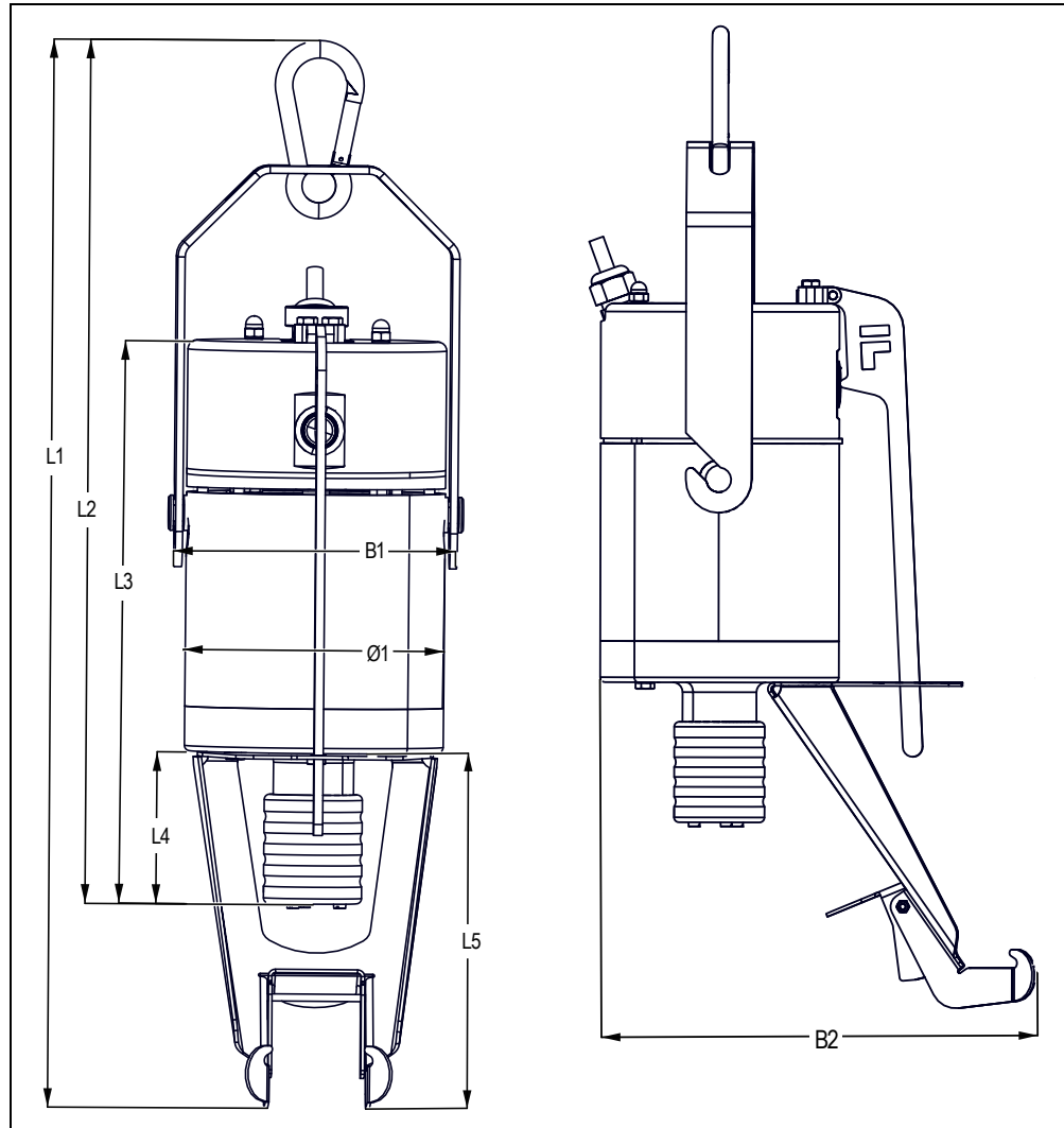
Fig. 3-6 Motor MDL1
