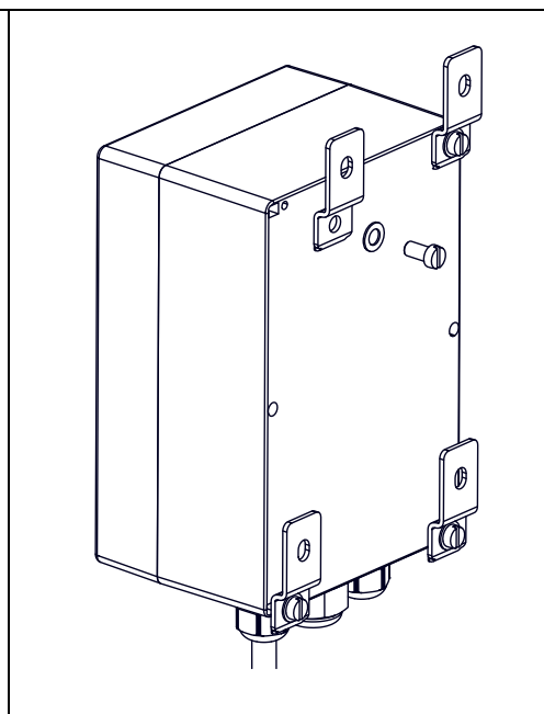
Рис. 5-5 ОпциональноДополнительно предлагаемый комплект для настенного монтажа, №-арт. 100-022-069
