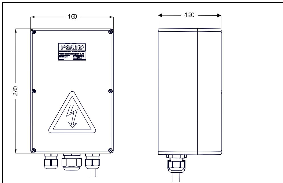
Рис. 3-12 Размеры управляющего устройства SG WBS51-08nc (в мм)
