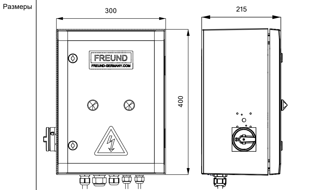
Рис. 3-10 Размеры управляющего устройства (указаны в мм)
