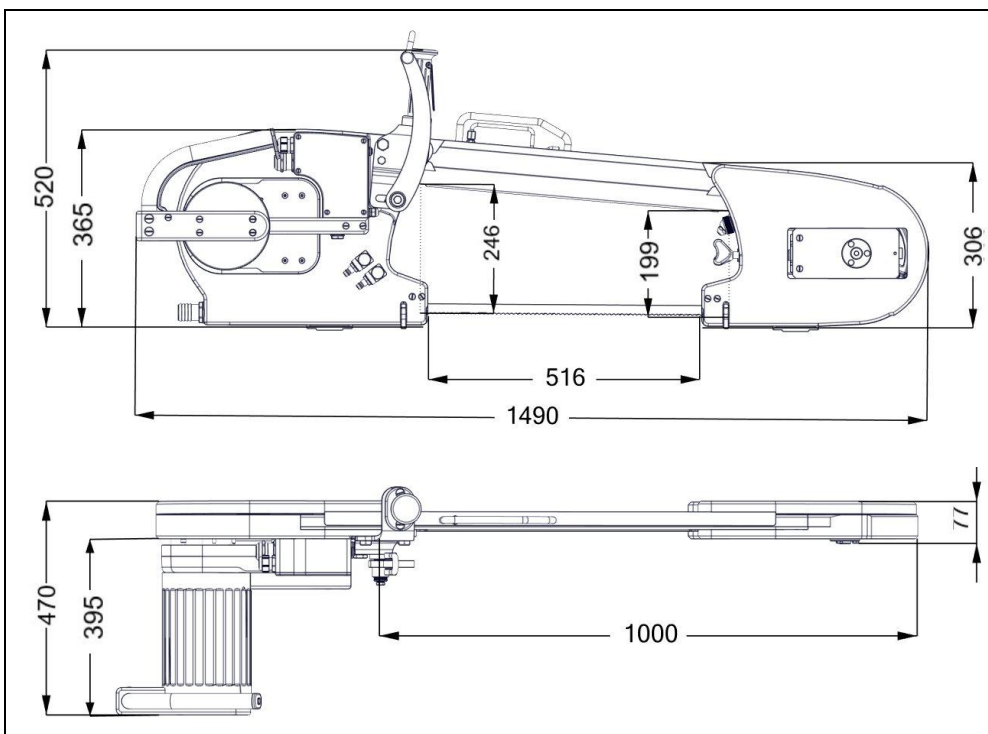
Рис. 3-3 Размеры WBS51-08 (в мм)
