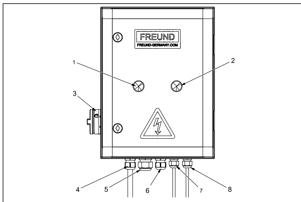
Рис. 3-9 Изображение управляющего устройства SG WBS51-08
