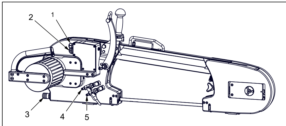
Рис. 3-6 Положение разъемов
