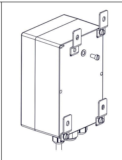
Rys. 5-5 Dostępny opcjonalny zestaw do montażu na ścianie, Nr-art. 100-022-069
