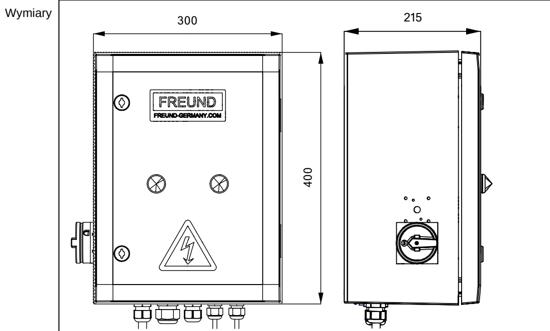
Rys. 3-10 Wymiary modułu sterującego (wymiary w mm)
