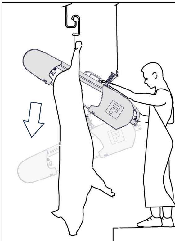
Rys. 6-1 Obsługa maszyny
