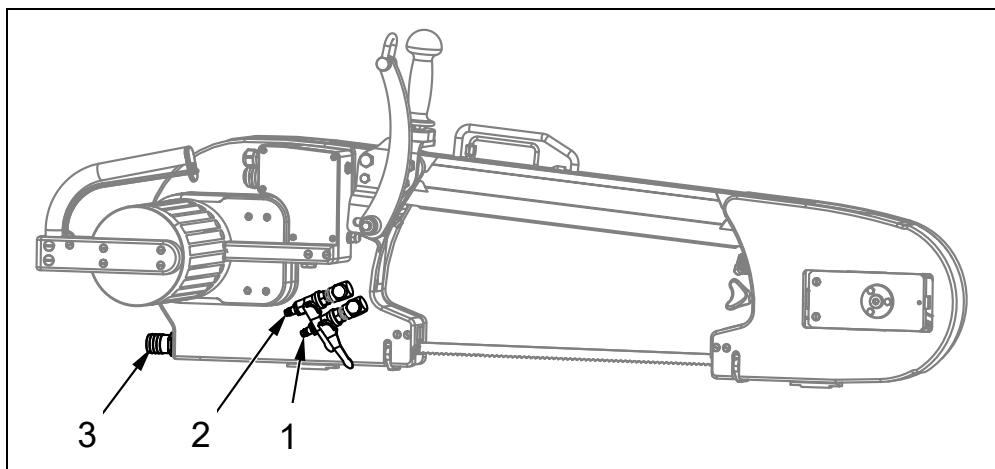
Rys. 5-9 Przyłącze wody
