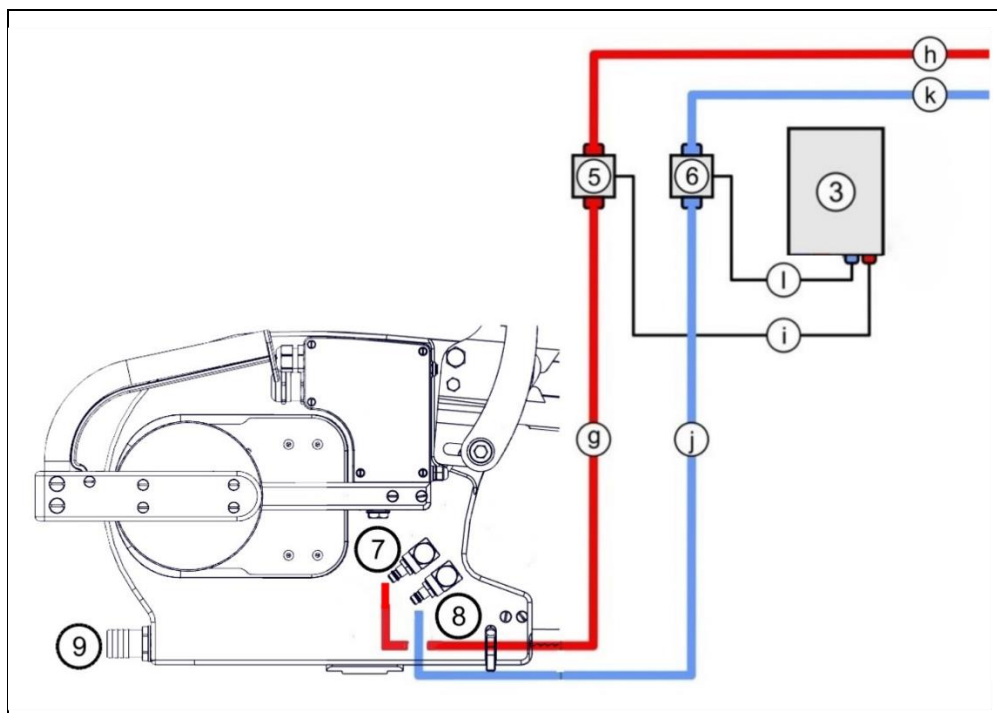
Rys. 5-7 Schemat przyłączy
