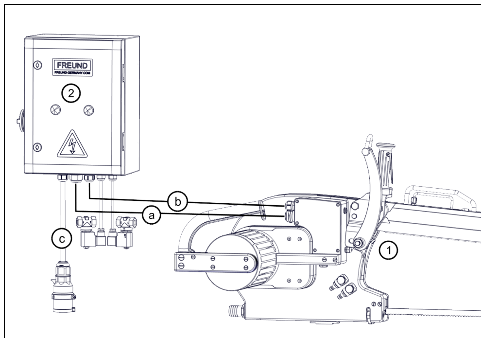
Rys. 5-6 Schemat przyłączy
