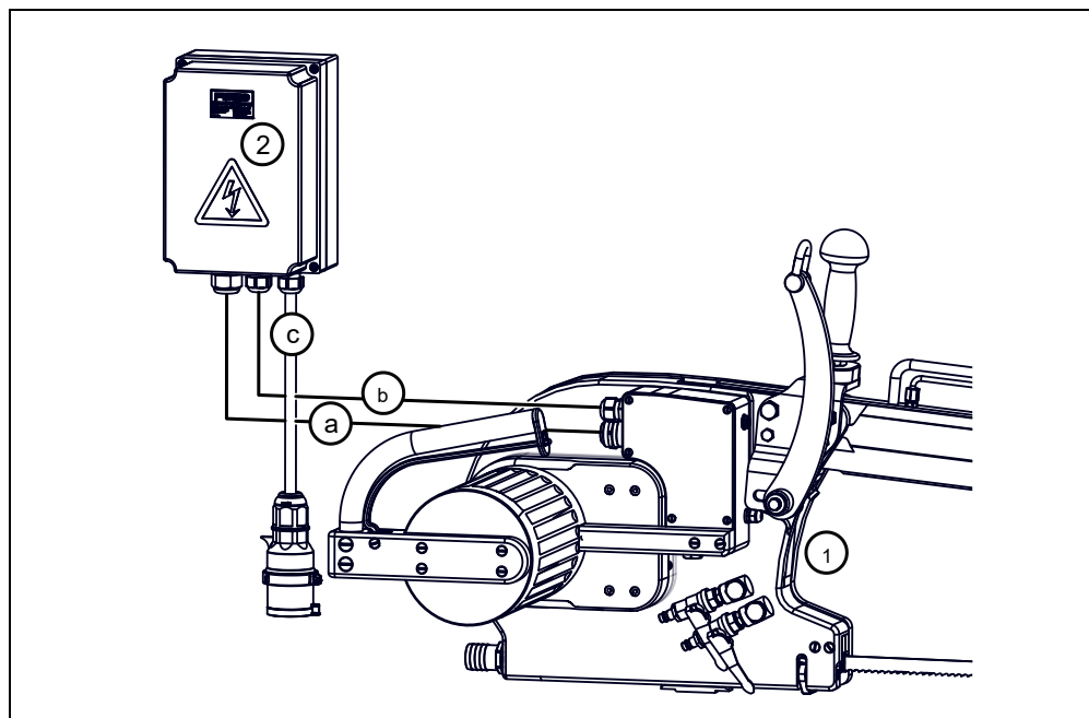
Rys. 5-8 Schemat przyłączy
