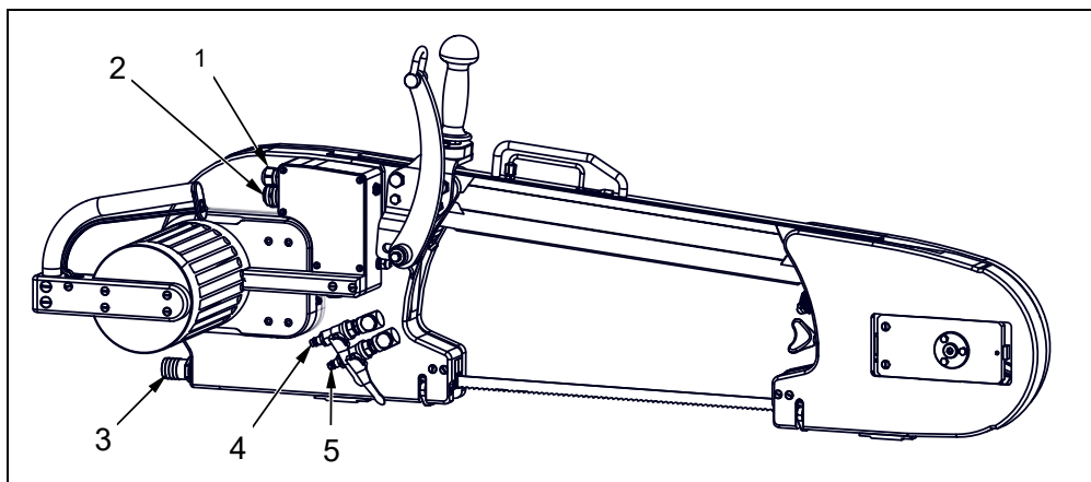
Rys. 3-6 Umiejscowienie przyłączy
