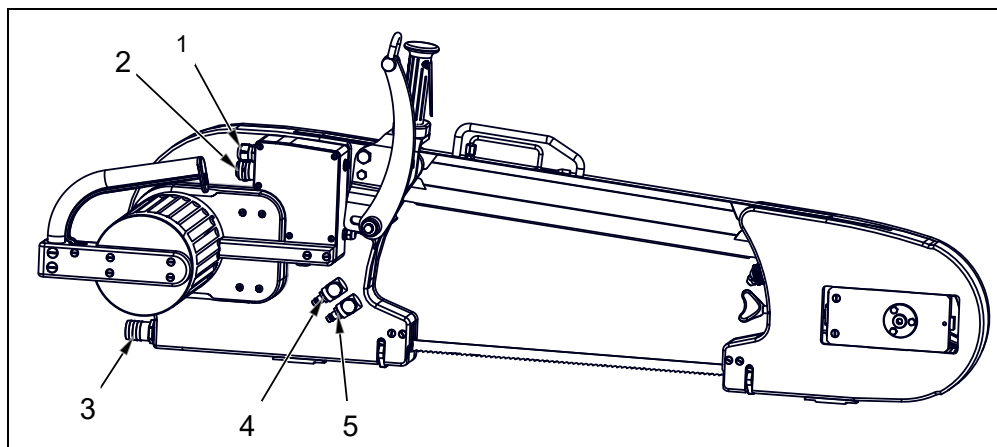
Rys. 3-2 Umieszczenie przyłączy
