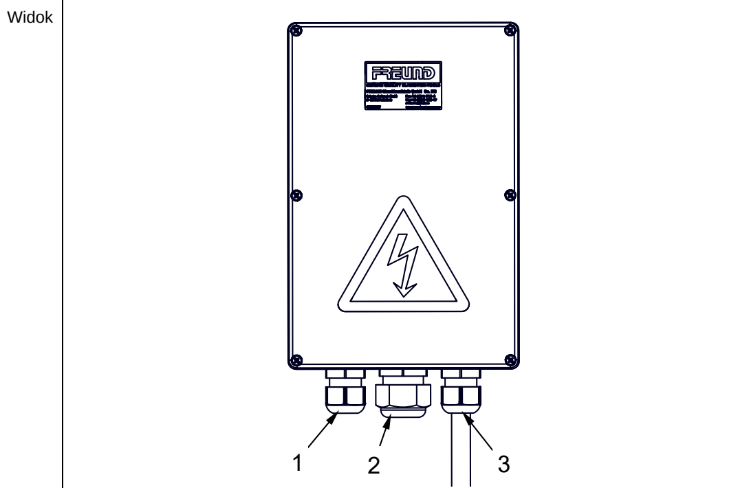
Rys. 3-11 Widok modułu sterującego SG WBS51-08nc
