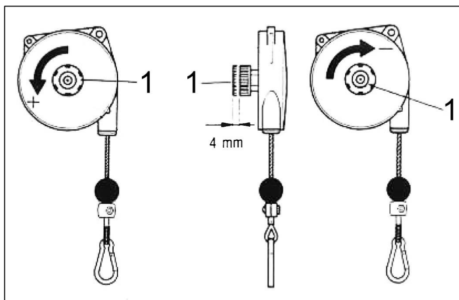
Рис. 5-2 Регулировка грузоподъемности
